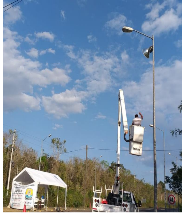
Instalación de luminaria tipo reflector en el filtro sanitario de Coba
