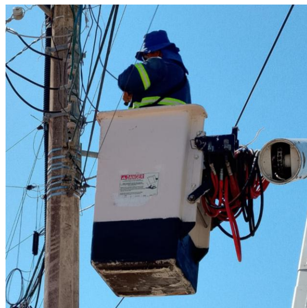
RECONEXIÓN DE LINEAS AEREAS PARA HABILITAR LUMINARIAS; POBLADO AKUMAL.
