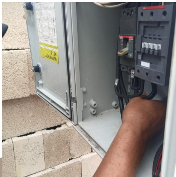
CAMBIO DE BASE DE FOTOCELDA PARA HABILITAR SECTOR; POBLADO COBA.
