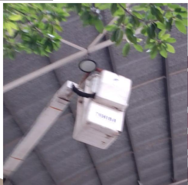
CAMBIO DE REFLECTORES FLAT; DOMO, UNIDAD DEPORTIVA, COL. CENTRO.
