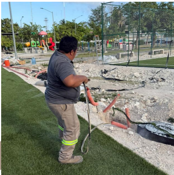
INSTALACIÓN DE LINEAS SUBTERRANEAS PARA HABILITAR LUMINARIAS; UNIDAD DEPORTIVA, COL. CENTRO.
