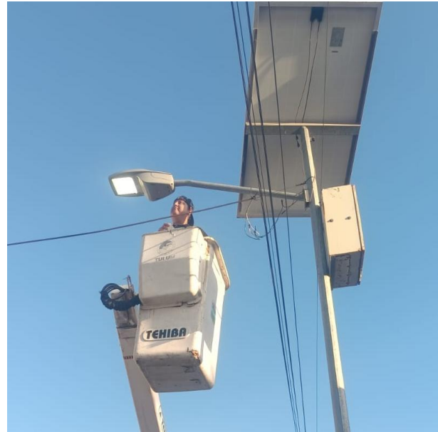
CAMBIO DE BASE Y FOTOCELDA OBSOLETOS POR NUEVOS; C. ALFA SUR ENTRE C. VENUS OTE Y C. NEPTUNO OTE, COL. CENTRO.
