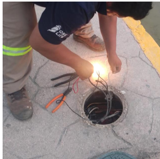
RECONEXIÓN DE LÍNEAS PARA HABILITAR LUMINARIAS; ZONA ARQUEOLOGICA.
