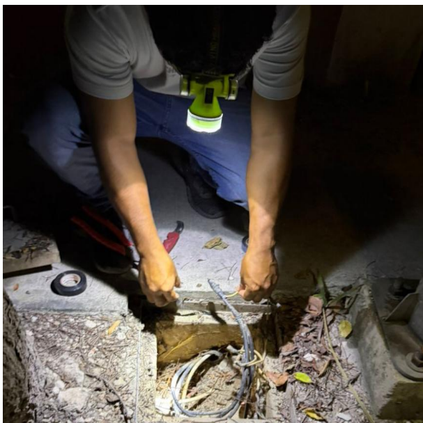
RECONEXIÓN DE LINEA SUBTERRANEA SULFATADA; PARA HABILITAR LUMINARIA; C. BUBULLEK ENTRE C. GEMINIS NTE Y C. LIBRA NTE, COL. MAYAPAX.
