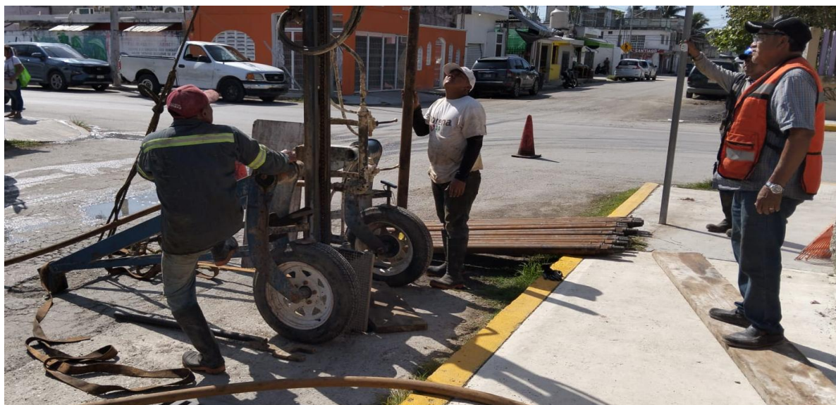
Desazolve. Av. 18 entre calle 19; colonia tumben kaa.
