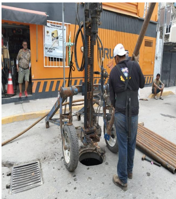
Desazolve. Av. Kukulkán entre calle mercurio poniente; colonia maya.
