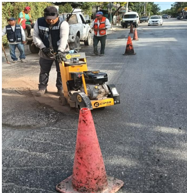
Bacheo. Av. kukulkán entre calle saturno norte y calle x-caret; colonia ejido.
