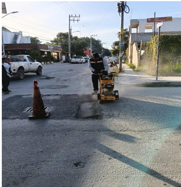
Bacheo. Calle alfa entre calle sagitario y calle polar; colonia centro.
