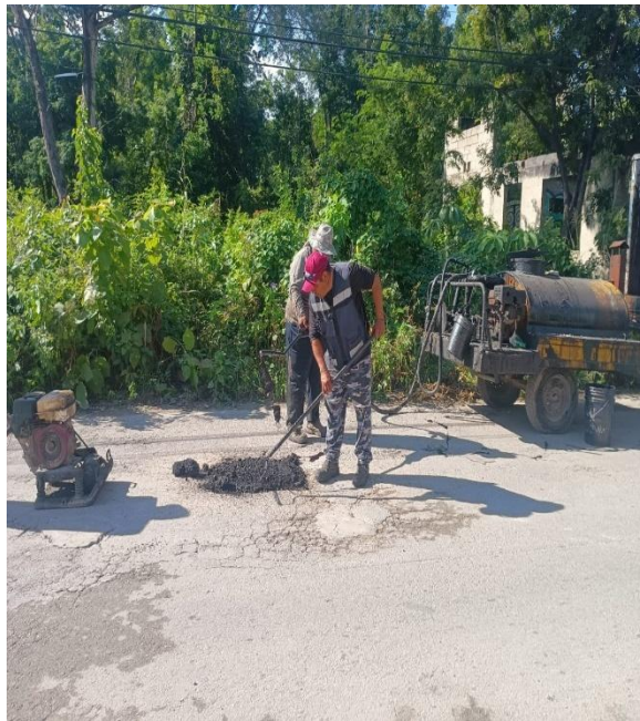
Bacheo. Calle zacil-ha entre calle chunyaxche y av. la selva; colonia ejido.
