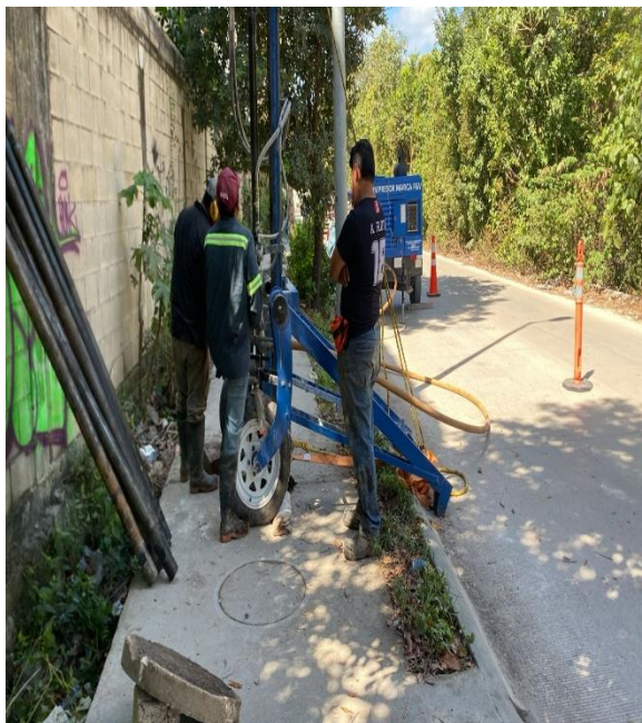
Desazolve. Calle juanek entre av. kukulkán y calle itzamna; fraccionamiento aldea zama.
