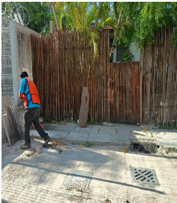
Limpieza de rejillas. Calle 2 bis oriente entre calle 11; fraccionamiento villas Tulum.
