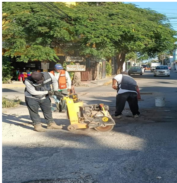
Bacheo. Calle tun-k'ul entre av. satélite; colonia mayapax.
