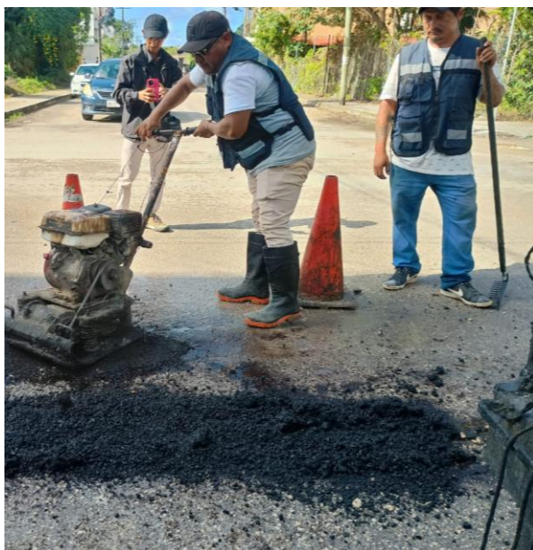
Bacheo. Av. Tulum entre calle acuario y calle luna; colonia centro.
