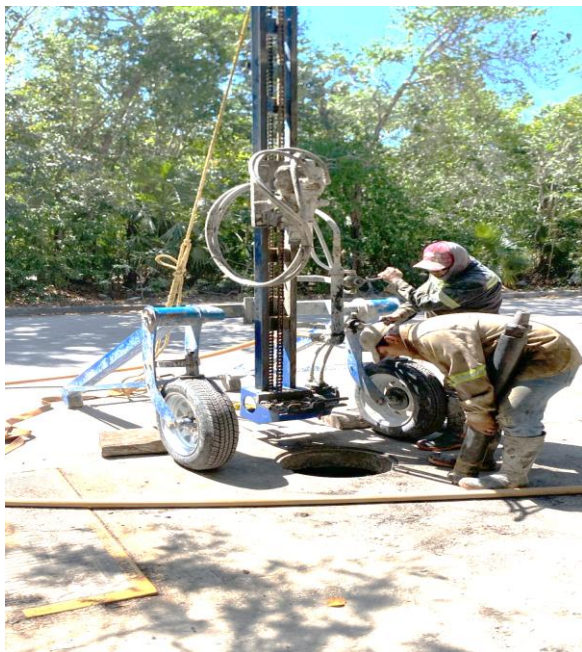
Desazolve. Av. cobá entre calle balam dzancab; fraccionamiento aldea zama. (Pozo 02).
