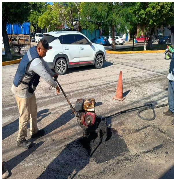
Bacheo. Calle andrómeda oriente entre av. satélite y calle géminis norte; colonia mayapax.
