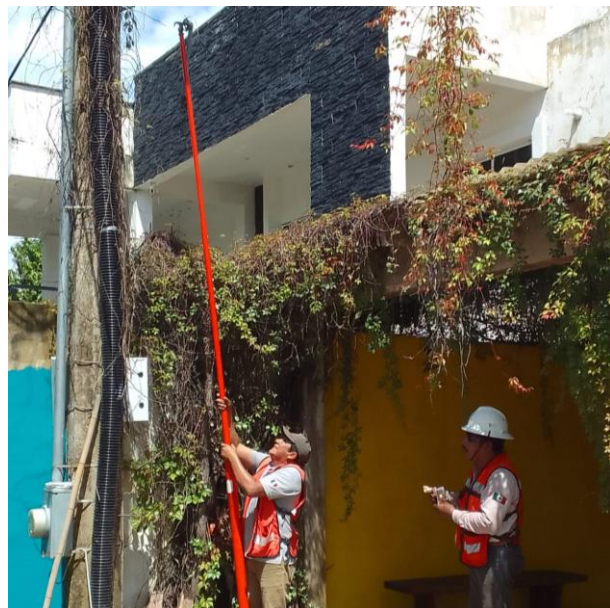
CAMBIO DE FUSIBLE A CUCHILLA; POBLADO FRANCISCO UH MAY.
