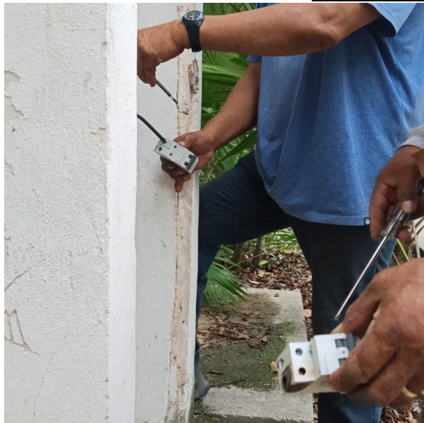
CAMBIO DE BREAK OBOSLETO POR NUEVO Y CAMBIO DE FOTOCELDA; FRACC. ALDEA ZAMA.
