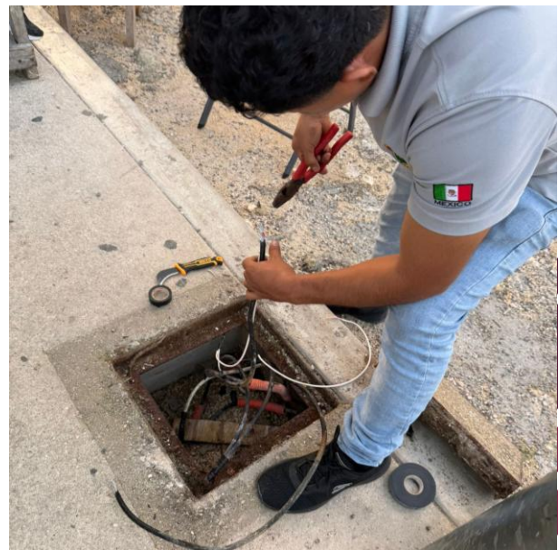
RECONEXIÓN DE LINEAS SUBTERRANEAS PARA HABILITAR LUMINARIAS; C. 27 ENTRE AV. YODZONOT Y CALLE 12, COL. TUMBEN-KAA.
