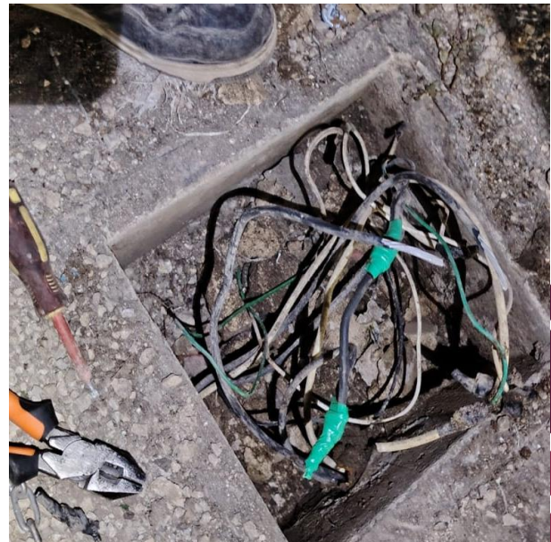
REVISIÓN Y RECONEXIÓN DE LINEAS SUBTERRANEAS SULFATADAS; AV. OSIRIS SUR ENTRE CALLE SOL, COL. CENTRO.
