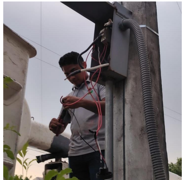
INSTALACIÓN DE CONTACTOR PARA AUTOMATIZAR SECTOR; CALLE 24 ENTRE 17, COL. TUMBEN-KAA.
