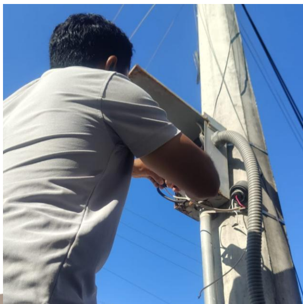
INSTALACIÓN DE CONTACTOR PARA AUTOMATIZAR SECTOR; CALLE 19 ENTRE CALLE 26, COL. TUMBEN-KAA.
