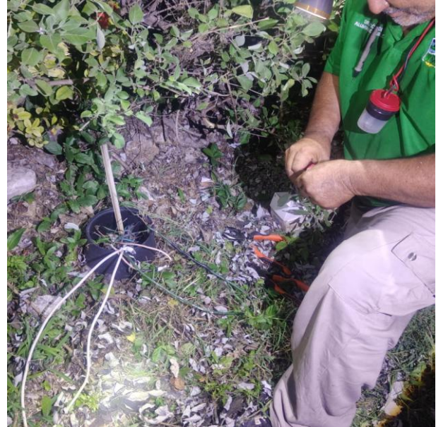
RECONEXIÓN DE LINEAS PARA HABILITAR REFLECTORES LED; UNIDAD DEPORTIVA, COL. CENTRO.
