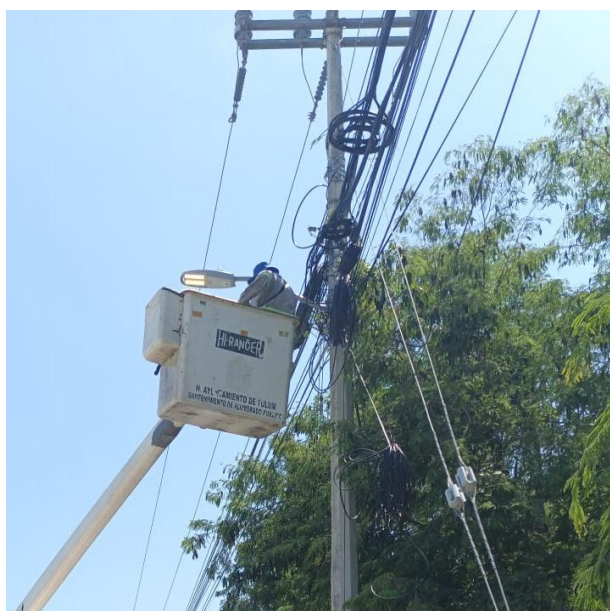
REPARACIÓN DE LAMPARA LED RECONECTANDO Y CAMBIANDO FOTOCELDA QUEMADA POR NUEVA; AV. OK-K'OOT ENTRE AV. COBA.
