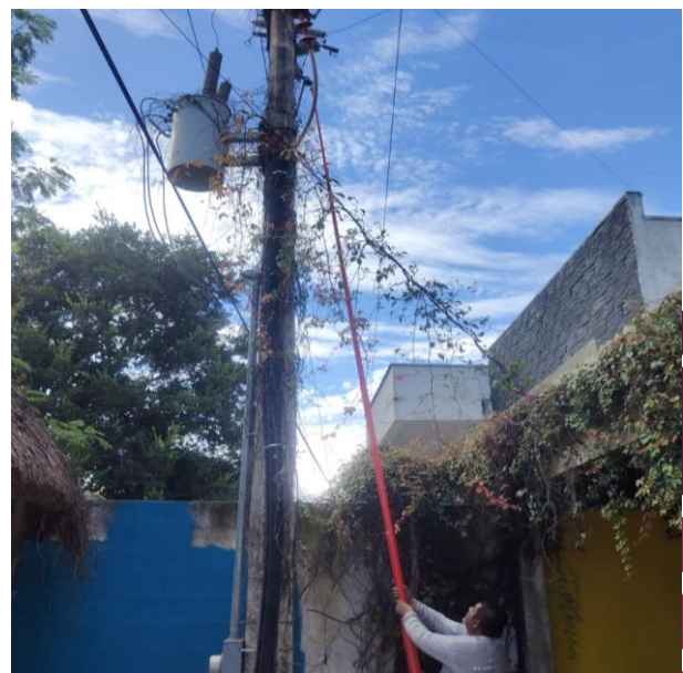
INSTALACIÓN DE FUSIBLES PARA CUCHILLAS PARA HABILITAR TRANSFORMADOR; POBLADO FRANCISCO UH MAY.
