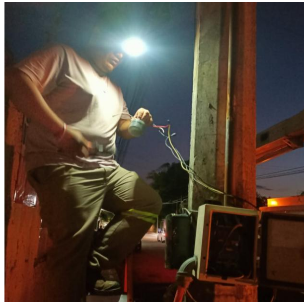
INSTALACIÓN DE BASE DE FOTOCELDA Y FOTOCELDA PARA HABILITAR SECTOR, CALLE CHAN-CHEN ENTRE CALLE GOLONDRINAS Y CALLE CALLINOLAS, COL. EJIDO.
