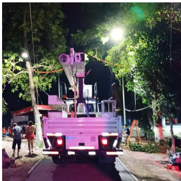
CAMBIO DE LUMINARIAS OBSOLETAS POR NUEVAS; UNIDAD DEPORTIVA, COL. CENTRO.
