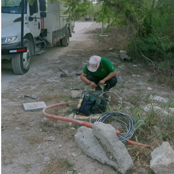
RECONEXIÓN DE LÍNEAS SUBTERRÁNEAS PARA HABILITAR LUMINARIAS; AV. 10 NTE, COL. MARITES.
