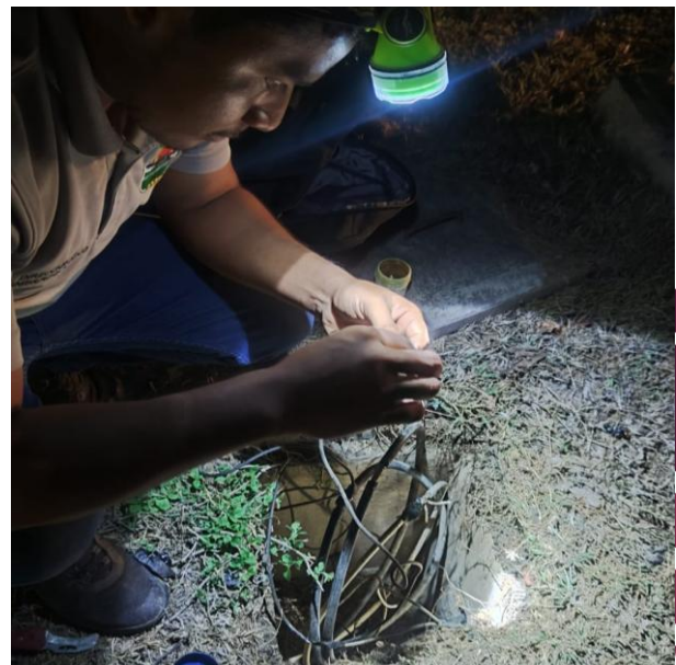
RECONEXIÓN DE LINEAS SUBTERRANEAS PARA HABILITAR LUMINARIAS; AV. TULUM.
