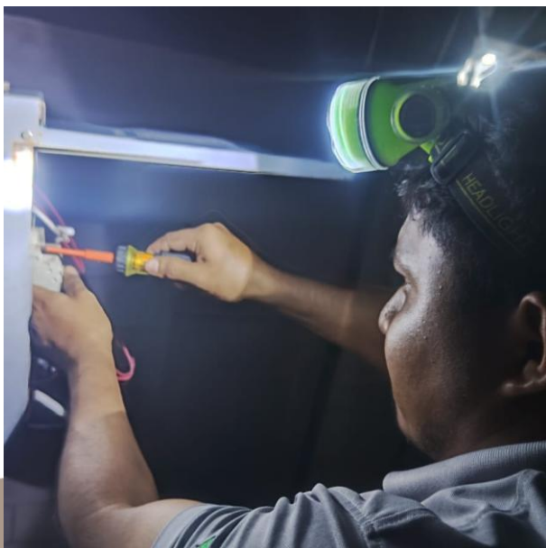
CAMBIO DE BASE DE FOTOCELDA Y FOTOCELDA, CALLE 24 ENTRE CALLE 17, COL. TUMBEN-KAA.
