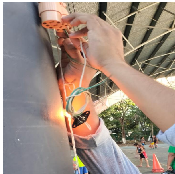
INSTALACIÓN DE BREAK Y CONTACTOR PARA AUTOMATIZAR SECTOR; CALLE 24, COL. TUMBEN-KAA.
