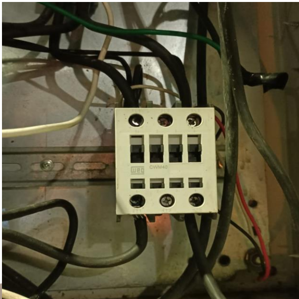
RECONEXIÓN DE LINEAS DE CONTACTOR PARA ACTIVAR LUMINARIAS, AV. OSIRIS SUR, COL. CENTRO.
