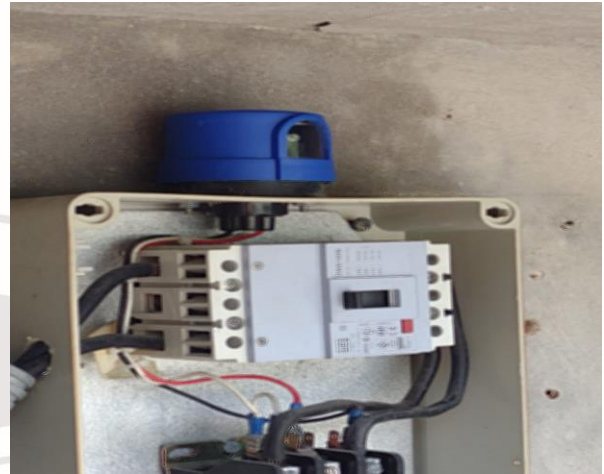
AKUMAL PUEBLO, REHABILITACIÓN DE BREAK DE 63WTS
