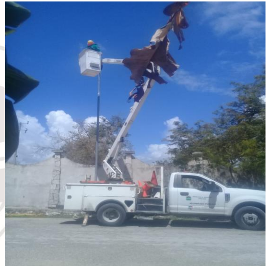
COL. TUBEN KA, AV. 28 / AV. 2 Y C. 27, SE REHABILITAN LAMPARAS Y BALASTROS OV-15 (TIPO AM-175W Y BALASTRO AM-175W)
