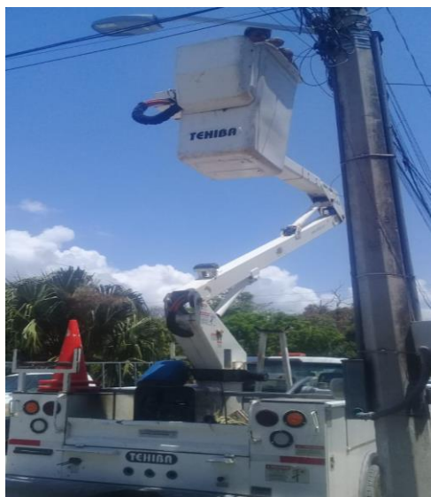
YAXCHE , REHABILITACIÓN DE LAMPARA OV-15 OBSOLETAS, CON LAMPARA LED DE 100 WATTS
