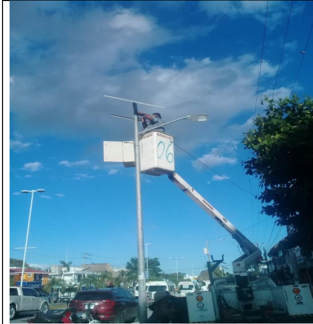
Rehabilitación de luminarias tipo led de driver colonia centro Av. Tulum Acuario Sur.
